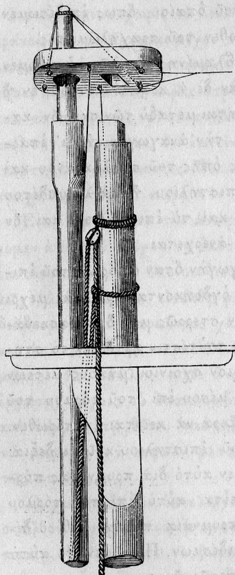
(Σ/. 146).—Τραχήλωσις τοῦ στηλοκράνου στήλης διὰ τοῦ μεγάλου ἐπιστηλίου.
