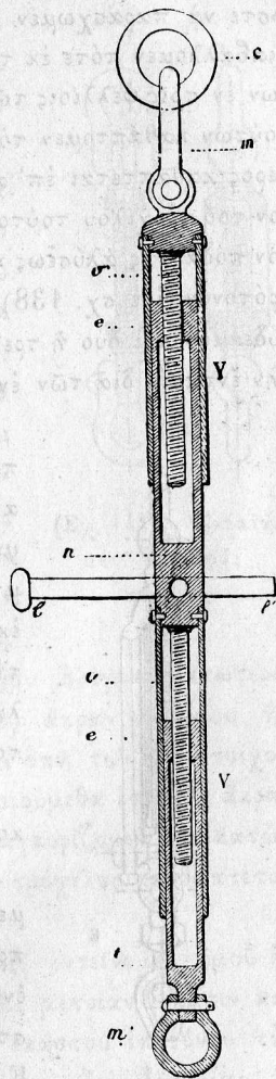
(Σχ. 139).—'Εντατήρ μετὰ σκεπαστοῦ κοχλίου.
