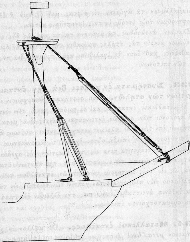
(Σχ. 138). — Πρόνευσις στήλης.
