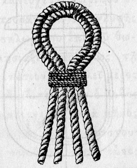
(Σχ. 150).—Διάταξις τραχηλώματος τῶν ἐπιτόνων μεγάλου ἐπιστηλίου κατὰ παρακύκλους.
