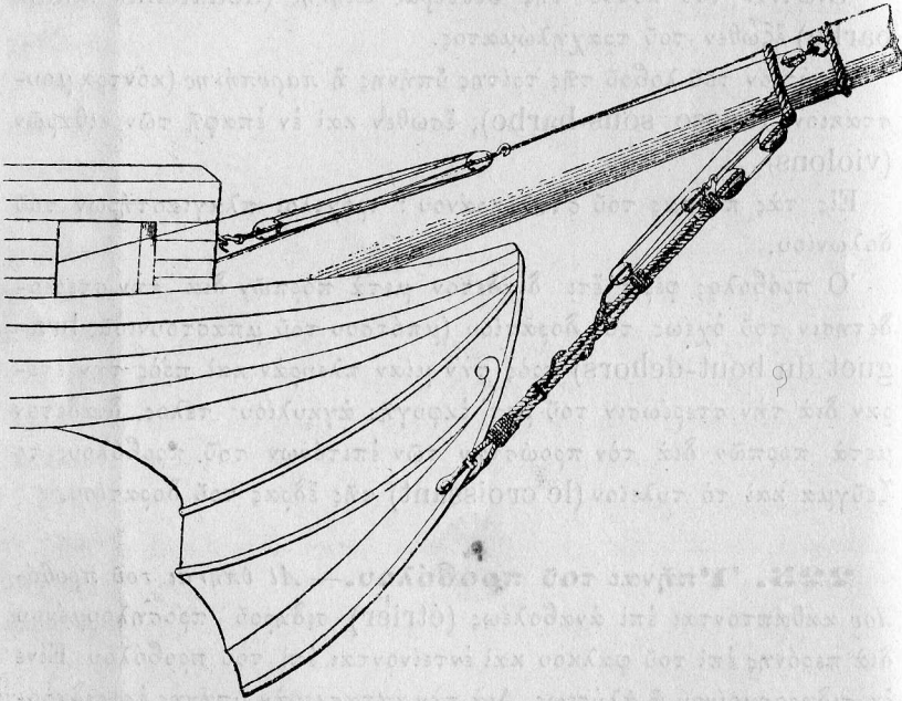
(Σγ. 136).—Ἐντασις ὑπῆνης.
