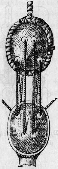
(Σχ. 142.)—Διαβολὴ ἐντονίου διὰ τῶν τετροπῶν.
