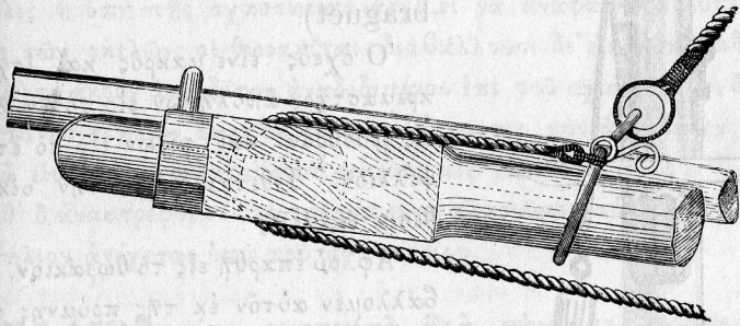
(Σχ. 153).— Ἀνάδρομος ἀρτέμονος μετὰ κορακιωτῆς κινητῆς στεφάνης.
