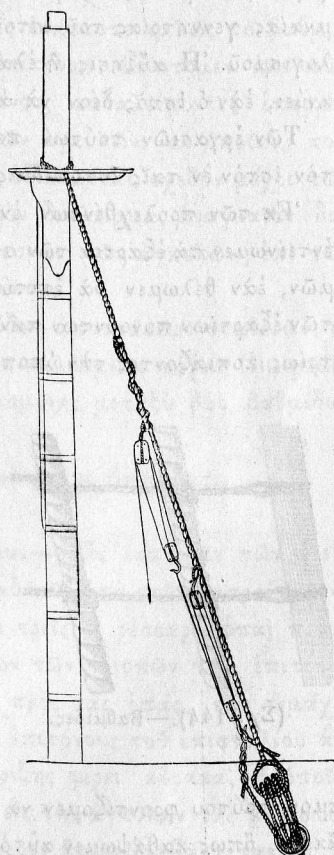
(Σελ. 143).—Ἐντασις κατωτέρου ἔξαρτιου (ἰχρυσύρτα).
