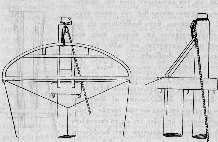
(Σχ. 149). — Τραχήλωσις διζύγων.
