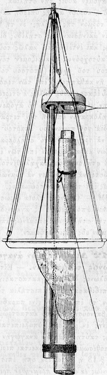
(Σ/. 147) — Τραχήλωσις τοῦ στηλοκράνου στήλης διὰ στηλίδος.
