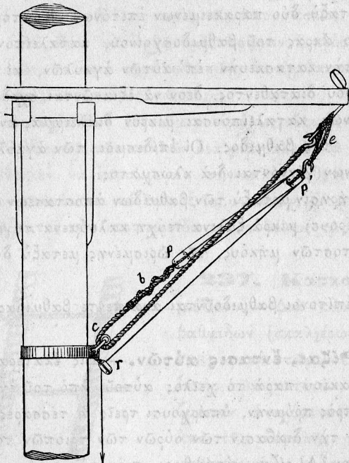
(Σ/. 145).—Ἐντασις ρίζης.
