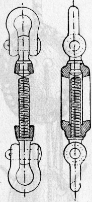
(Σχ. 141).—Ἐντατήρ μετ' ἀσκεποῦς κοχλίου.
