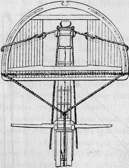
(Σ/. 133).—Τραγήλωσις θωρακίου.
