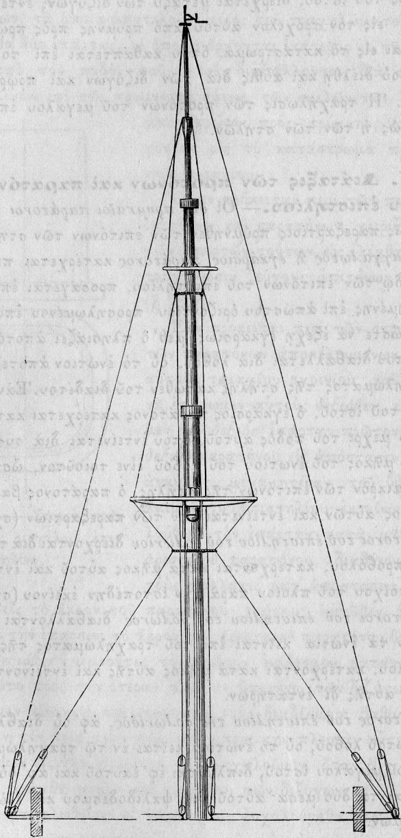
(Σχ. 152). — Διάταξις τῶν παρατόνων τῶν μεγάλων καὶ μικρῶν ἐπιστηλίων.
